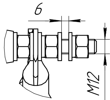
Б(1:2) Подключение ВН
