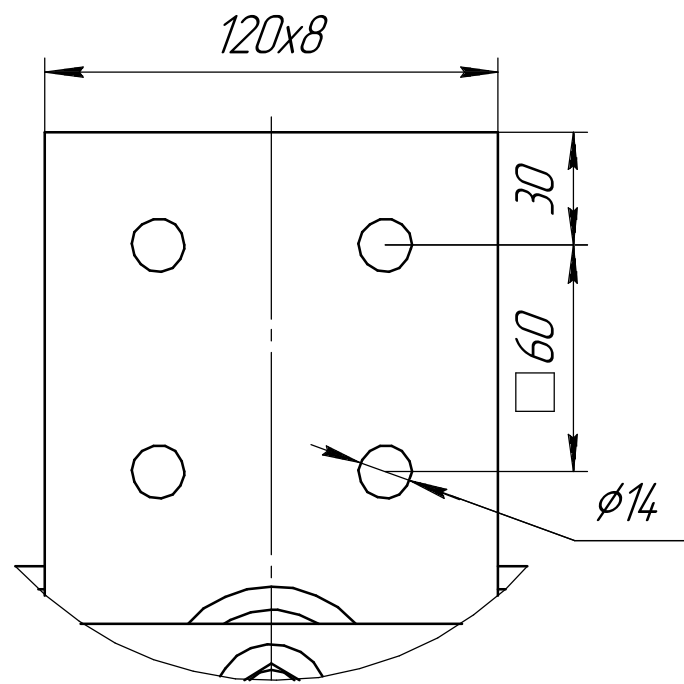
А(1:2) Подключение НН
