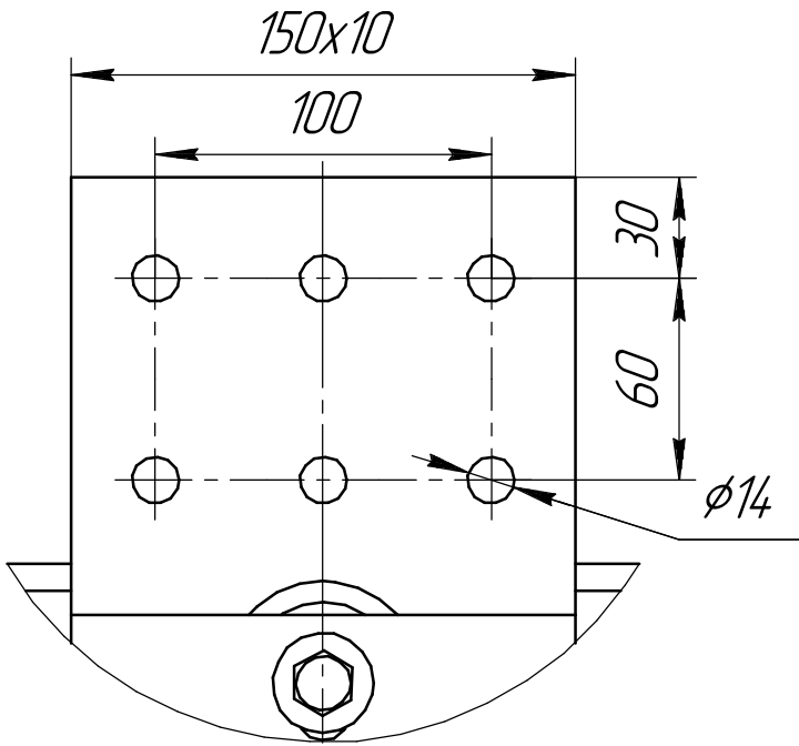
А(1:2,5) Подключение НН
