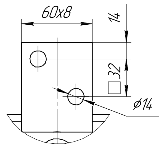
А(1:2) Подключение НН
