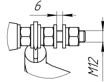
Б(1:2) Подключение ВН
